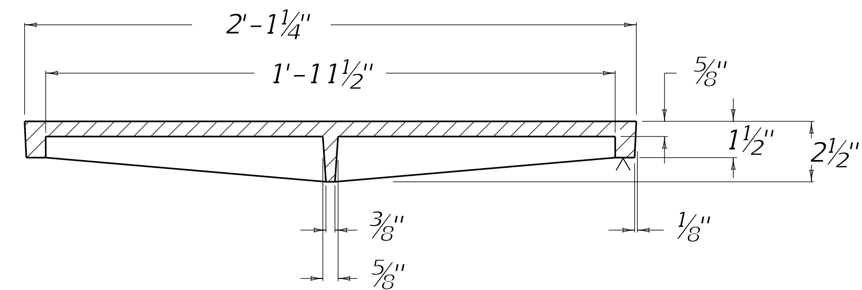
SECTION A-A
